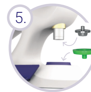
5. Werkzeug-Set für Ösen einlegen.
